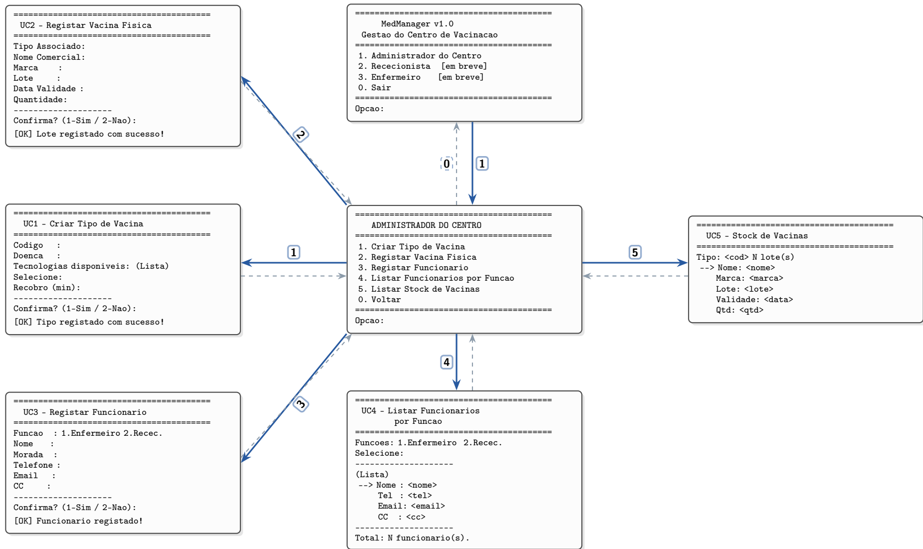
Figure 1: User Interface Design – Diagrama de Fluxo de Ecrãs (CLI), Ator: Administrador do Centro. Setas a cheio (→) representam navegação de entrada; setas a tracejado representam retorno ao menu anterior.
